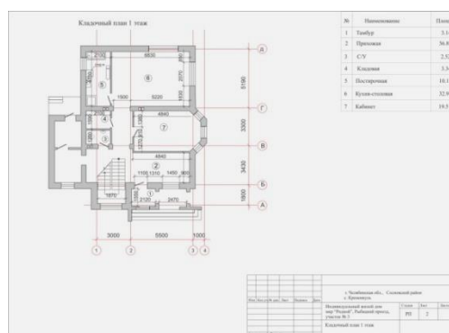
Рис. 1. План 1 этажа
